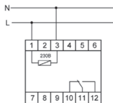
Схема подключения PCU-511/PCU-511U
