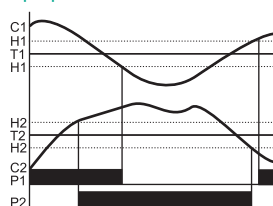
Программа 5. Охлаждение
