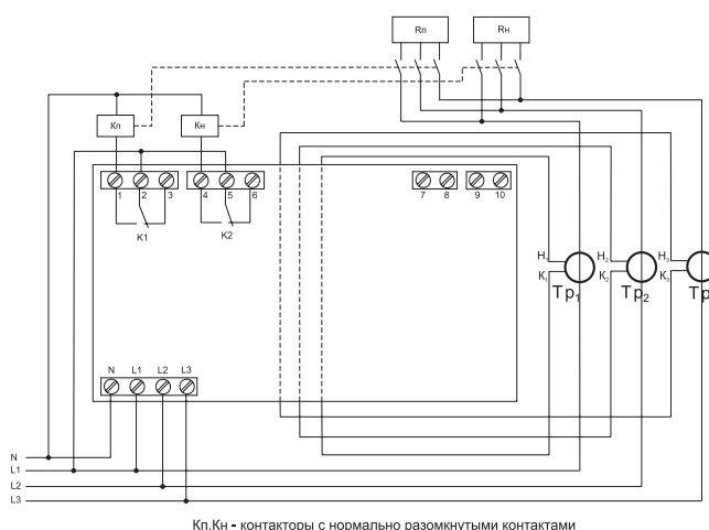
Схема включения OM-630-2
