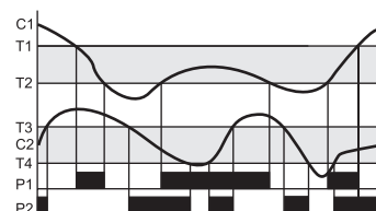
Программа 10. Работа в режиме «Два окна» по температуре C1 и C2
