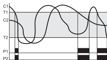
Программа 9. Работа в режиме «Окно» по температуре C1 и C2
