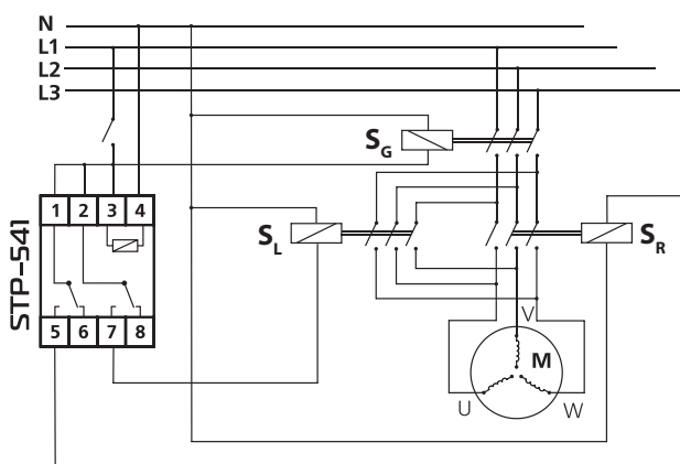
S_G – основной контактор; S_R и S_L – контакторы переключения фаз
