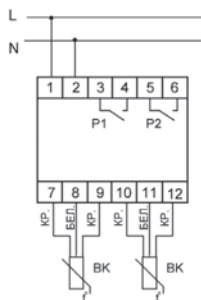
Программа 1. Нагрев
