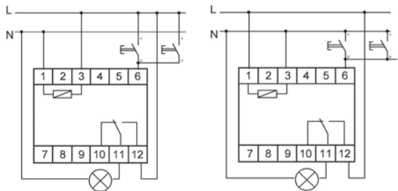
Кнопки управления подключены к фазному проводу L
