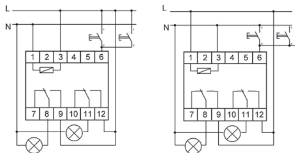
Кнопки управления подключены к фазному проводу L
