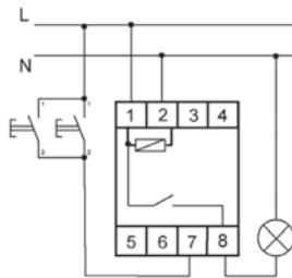
С функцией предупреждения о выключении и антиблокировкой
