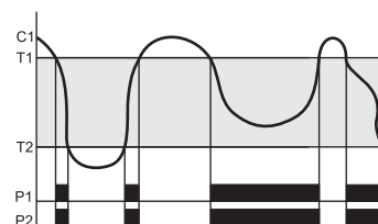
Программа 8. Работа в режиме «Окно»
